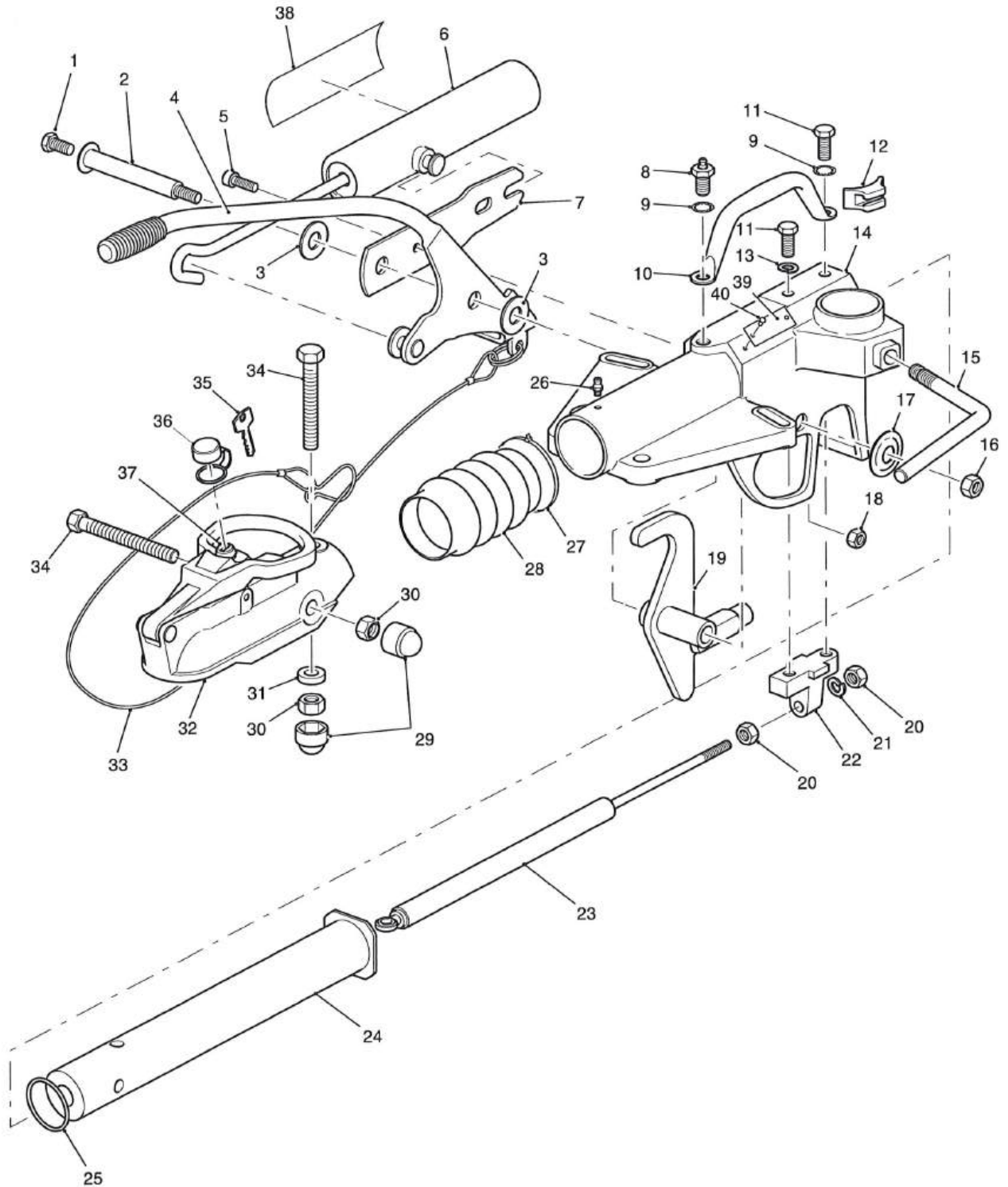
COUPLING KFG27
